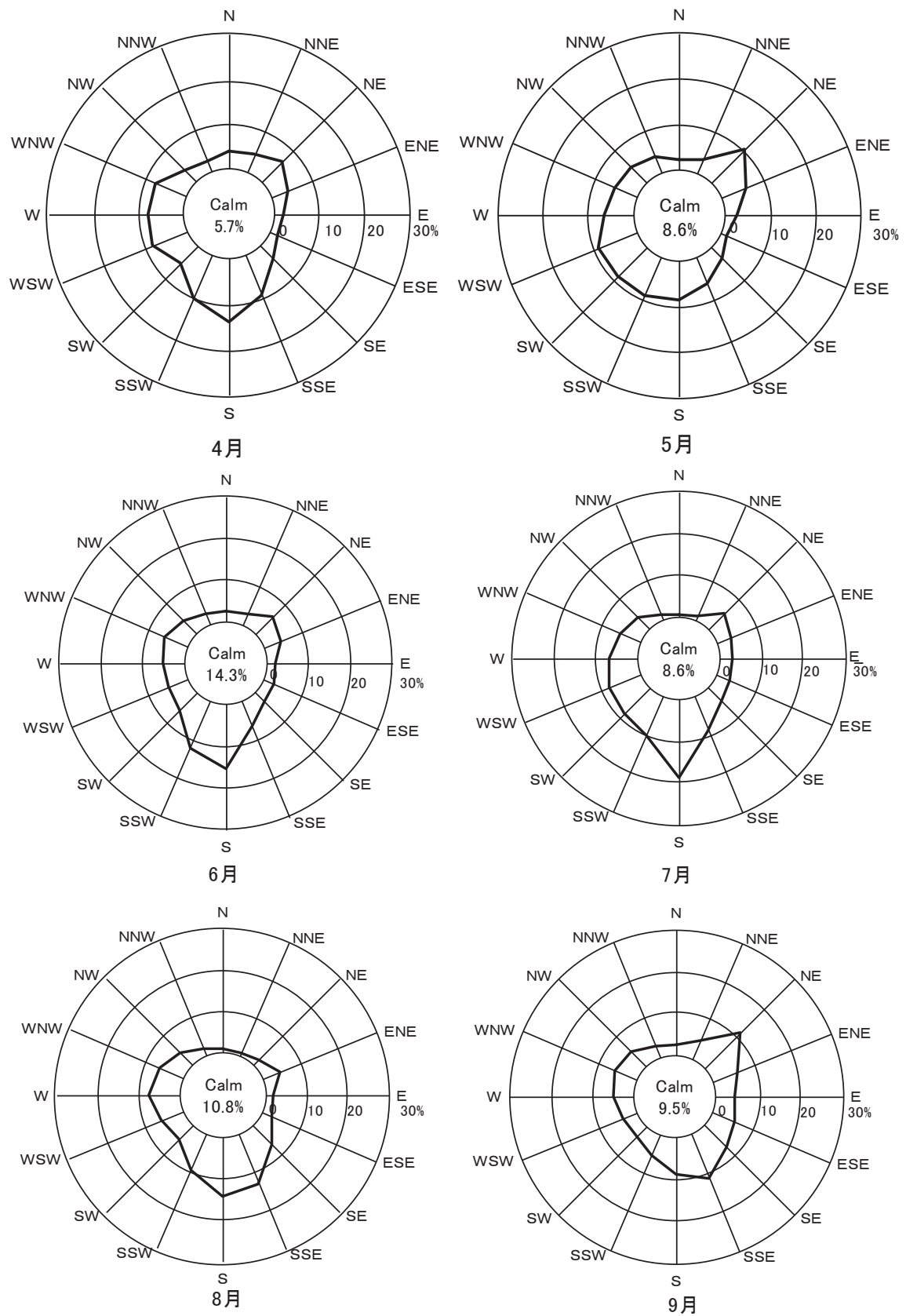
図Ⅲ. 2. 2(1) 泉佐野市日根野浄水場局風配図
