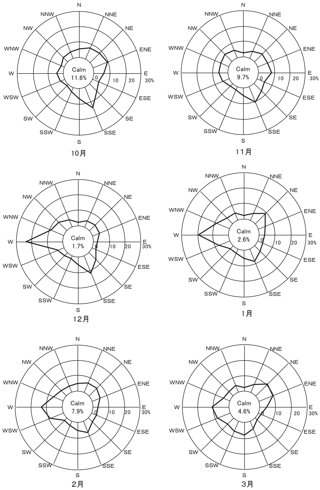
図Ⅲ.2.2(2) 泉佐野市日根野浄水場局風配図
