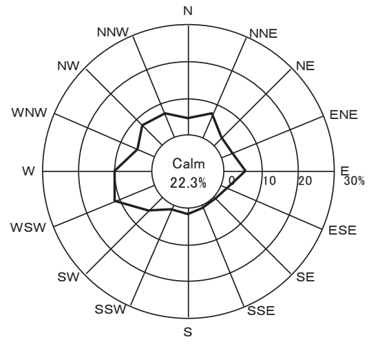
図Ⅲ.2.3(1) 近畿大学グランド局風配図
