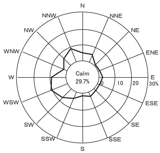
図Ⅲ.2.3(1) 近畿大学グランド局風配図
